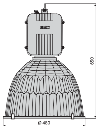
DUSTRA 480RM
